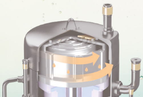
Перший ступінь сепарації
