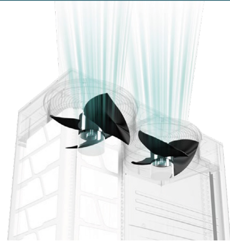
Високоефективний осьовий вентилятор
