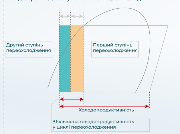
P-h діаграма двоступеневого переохолодження
