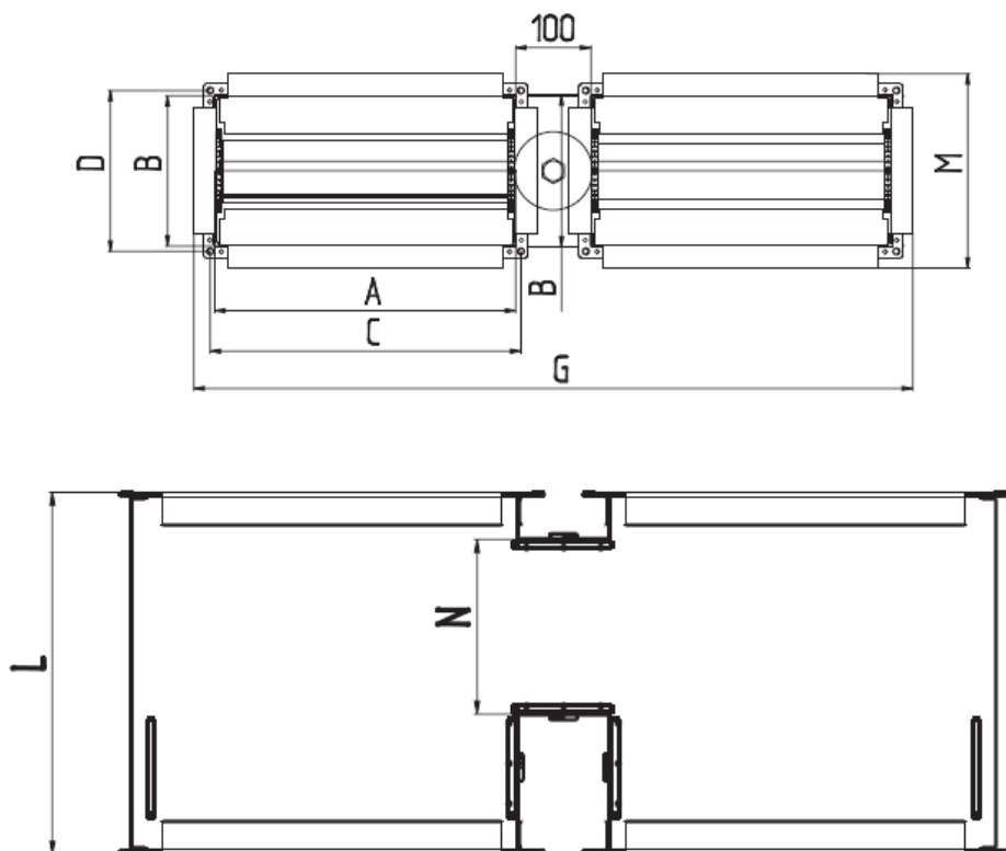
Рис 2 – Габаритні та приєднувальні розміри
