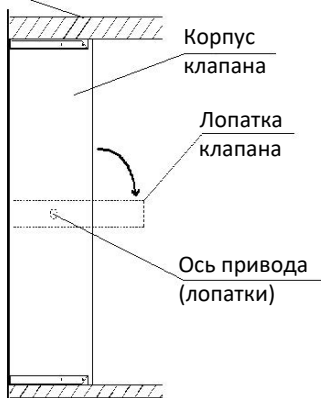
Строительная конструкция с носмированным пределом огнестойкости
