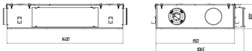
Рис 7. Габаритні розміри SlimStar 500
