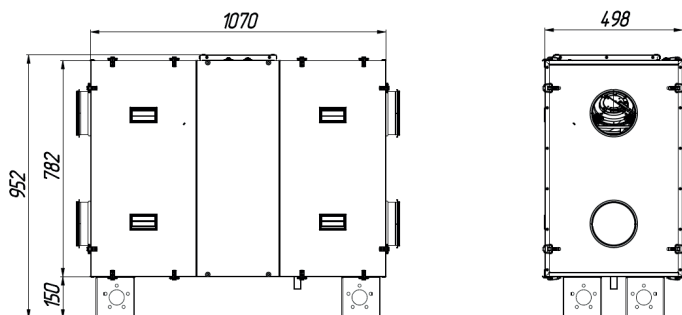
Рис 2. Габаритні розміри EcoStar 500X
