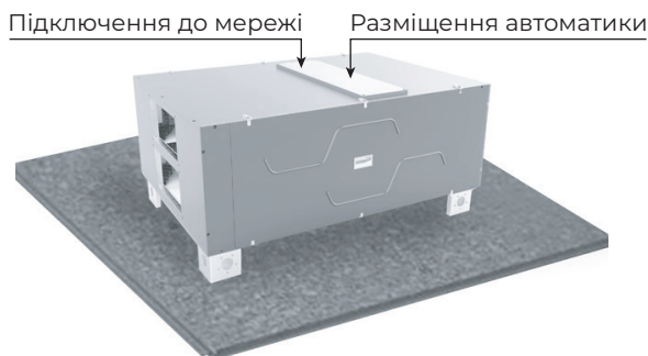
Рис. 24 Розміщення установки
