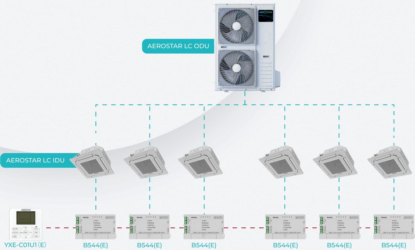
Схема демонструє приклад з'єднання зовнішнього блоку серії AEROSTAR LC із шістьма внутрішніми касетними блоками.
