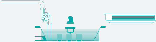
2 Коли дренажний насос перестає працювати, а рівень води підвищується завдяки великій конструкції зливного піддону, кондиціонер продовжує працювати в нормальному режимі.
