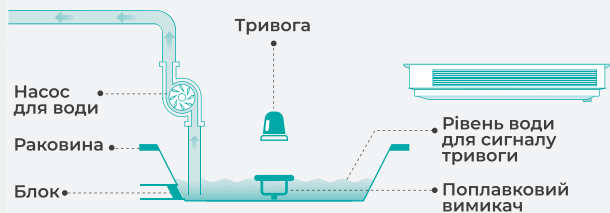
1 Датчик рівня води
