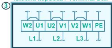
Клемна коробка / Terminal box
