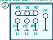
Υ Схема / Scheme 400 V більше 2.2 кВт / more than 2.2 kW
