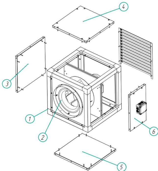
Рисунок 3 Конструкція вентилятора
