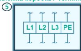
Клемна коробка / Terminal box
