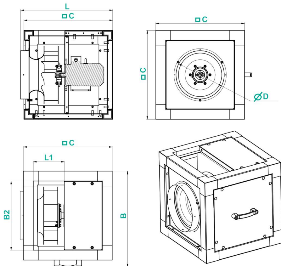
Рисунок 1 Габаритні розміри KFS
