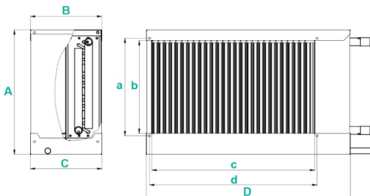
Рисунок 1 - Габаритні та приєднувальні розміри
